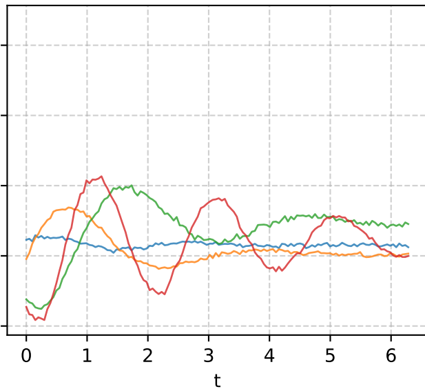
Diffusion
